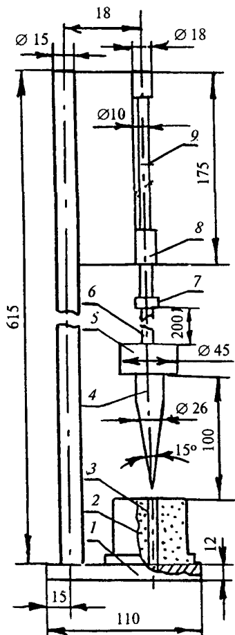
Рисунок 13 — Прибор для определения слеживаемости
