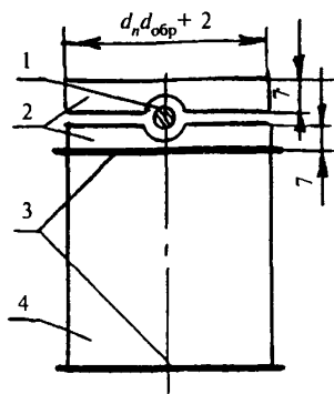
Рисунок 6 — Шарнирное устройство
