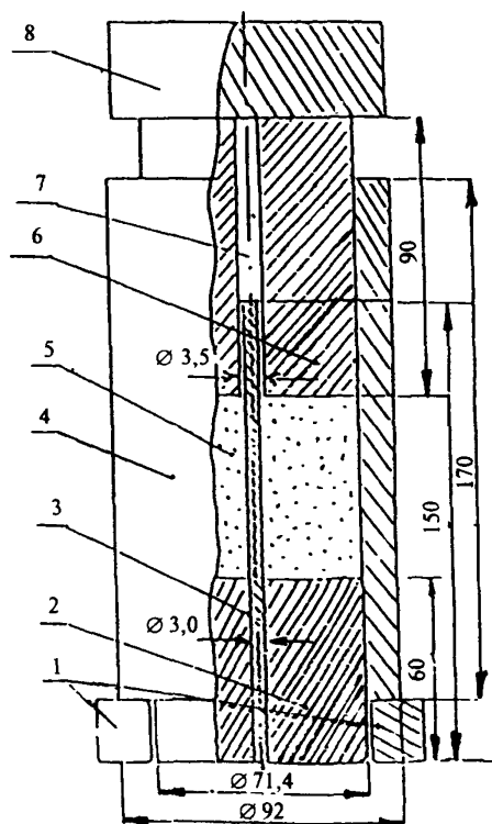
Рисунок 3 — Приспособление для уплотнения образцов из холодных смесей для определения слеживаемости
