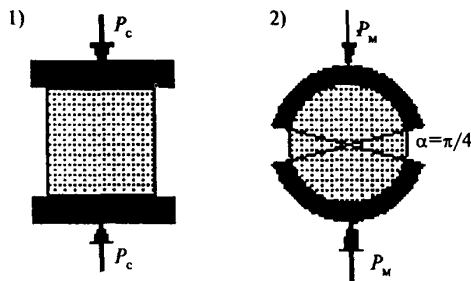
Рисунок 9 — Схема испытания образцов на сдвигустойчивость
